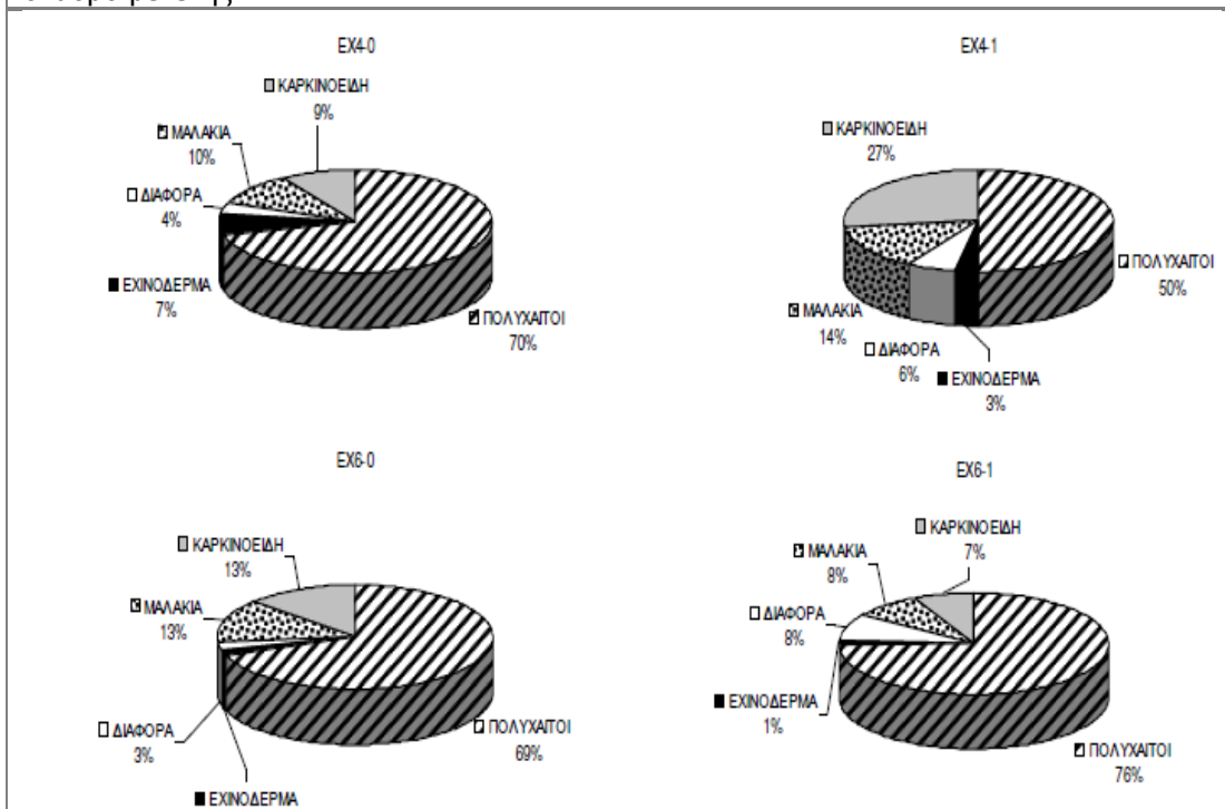
Διάγραμμα 6.10 Ποσοστιαία σύσταση των κύριων ομάδων στη συνολική αφθονία για κάθε σταθμό μελέτης.
