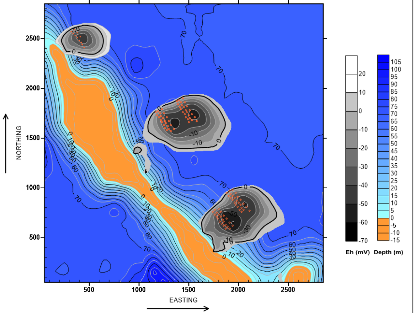
Διάγραμμα 7.84 Μεταβολή δυναμικού οξειδοαναγωγής του ιζήματος (Π1 – Σενάριο 4).
