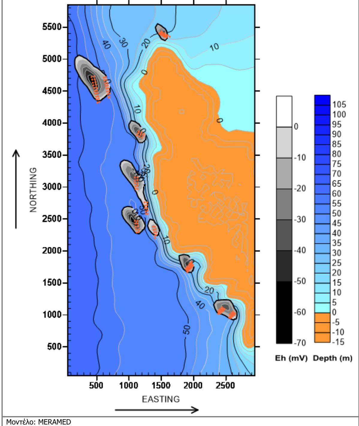
Διάγραμμα 7.39 Μεταβολή δυναμικού οξειδοαναγωγής του ιζηματος (Π3 – Σενάριο 2).
