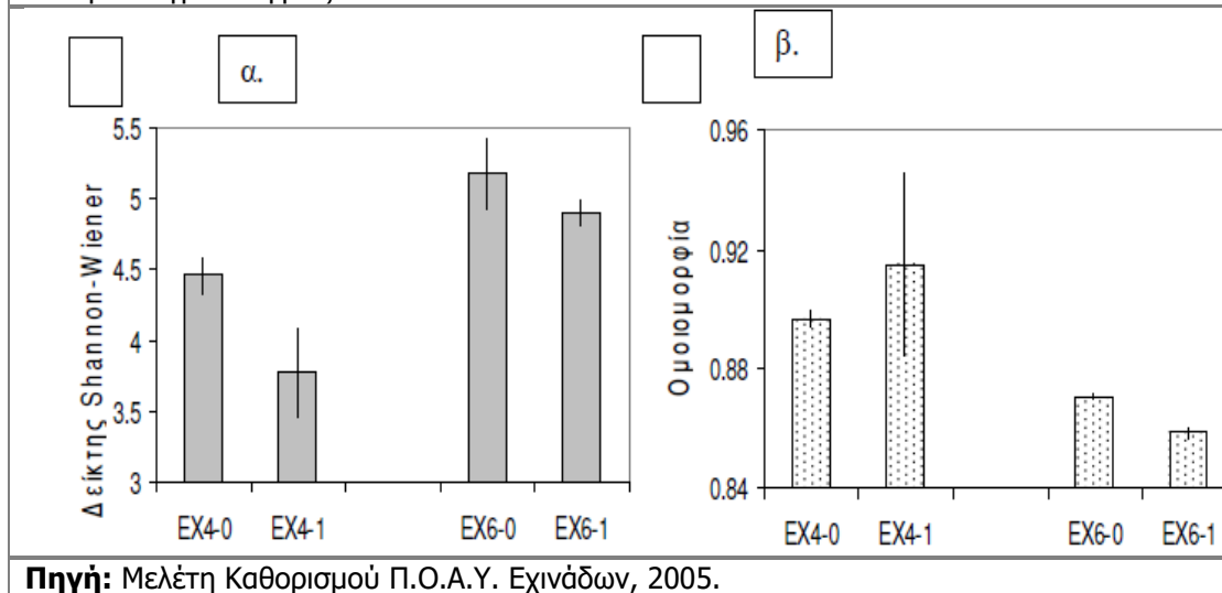
Διάγραμμα 6.9 Δείκτες α) ποικιλότητας Shannon-Wiener και β) ομοιομορφίας Pielou, ανά σταθμό δειγματοληψίας.
