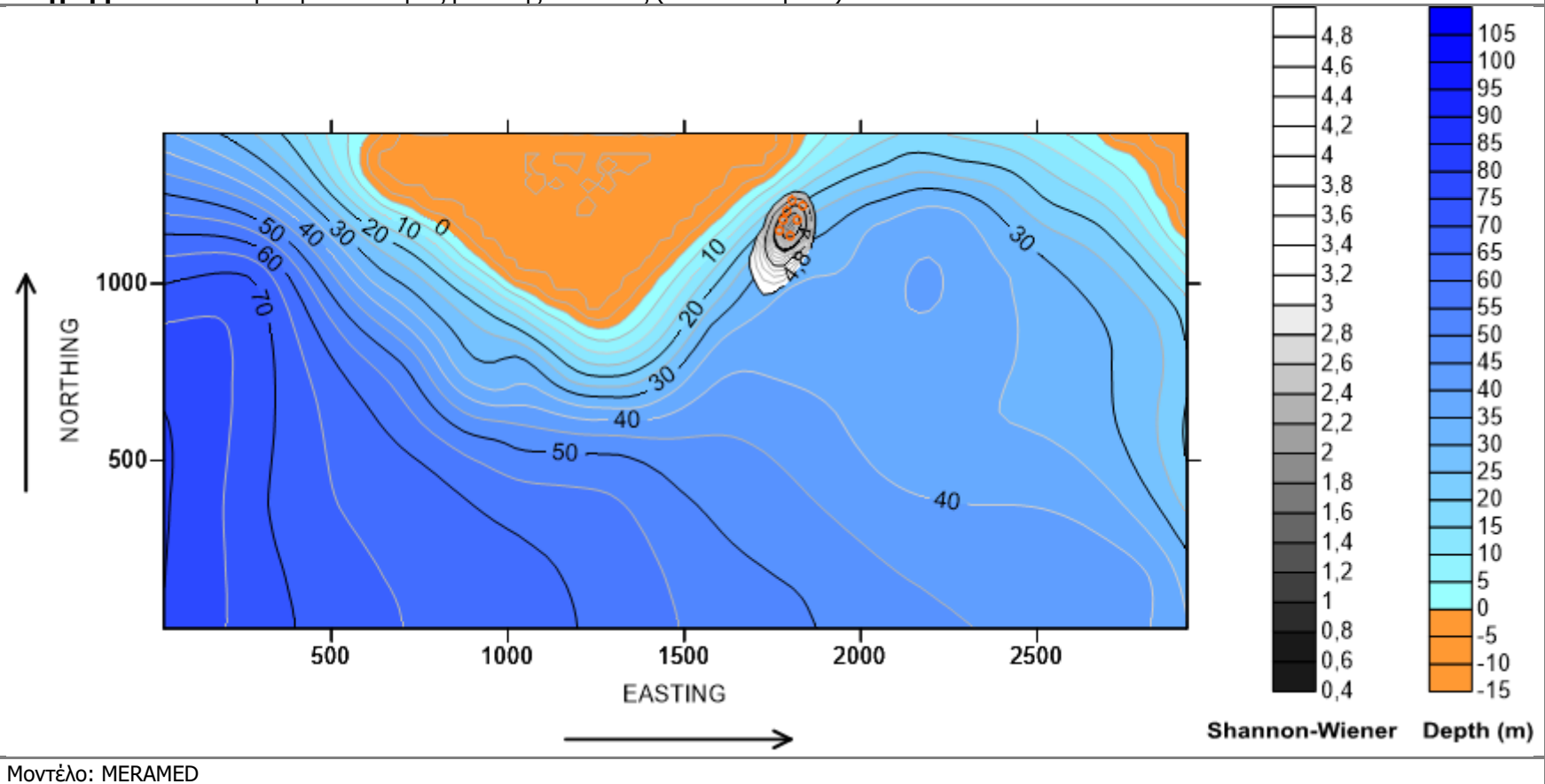
Διάγραμμα 7.59 Μεταβολή ποικιλότητας βενθικής κοινότητας (Π10 – Σενάριο 2).
