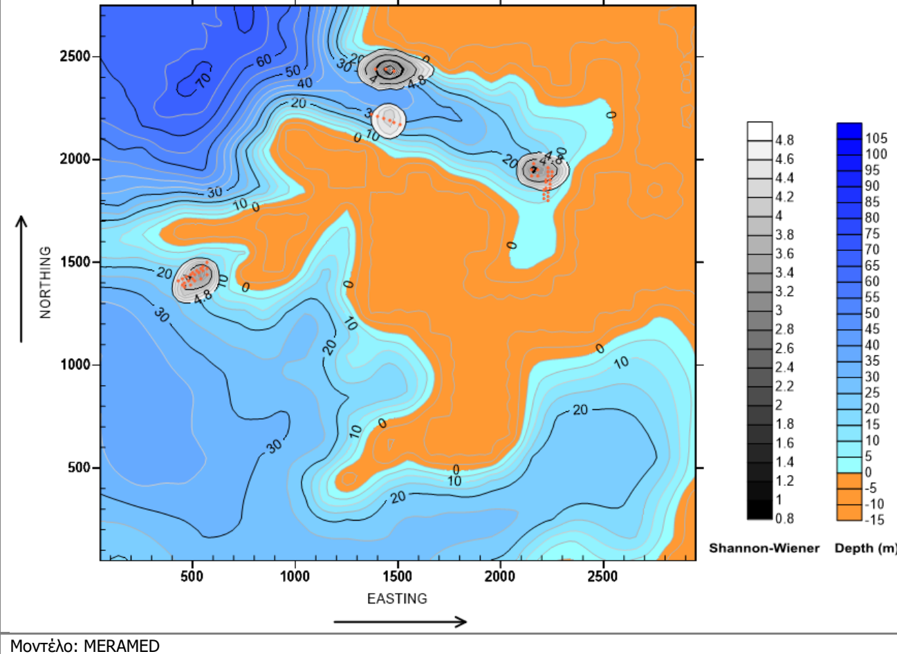
Διάγραμμα 7.14 Μεταβολή ποικιλότητας βενθικής βιοκοινωνίας (Π5- Σενάριο 1).
