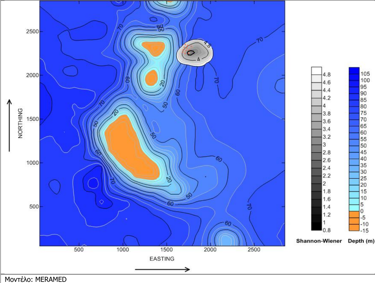
Διάγραμμα 7.23 Μεταβολή ποικιλότητας βενθικής βιοκοινωνίας (Π8- Σενάριο 1).
