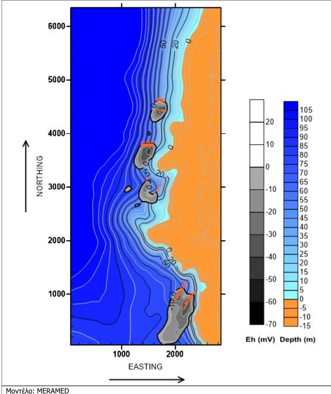
Διάγραμμα 7.99 Μεταβολή δυναμικού οξειδοαναγωγής του ιζήματος. (Π6 – Σενάριο 4).
