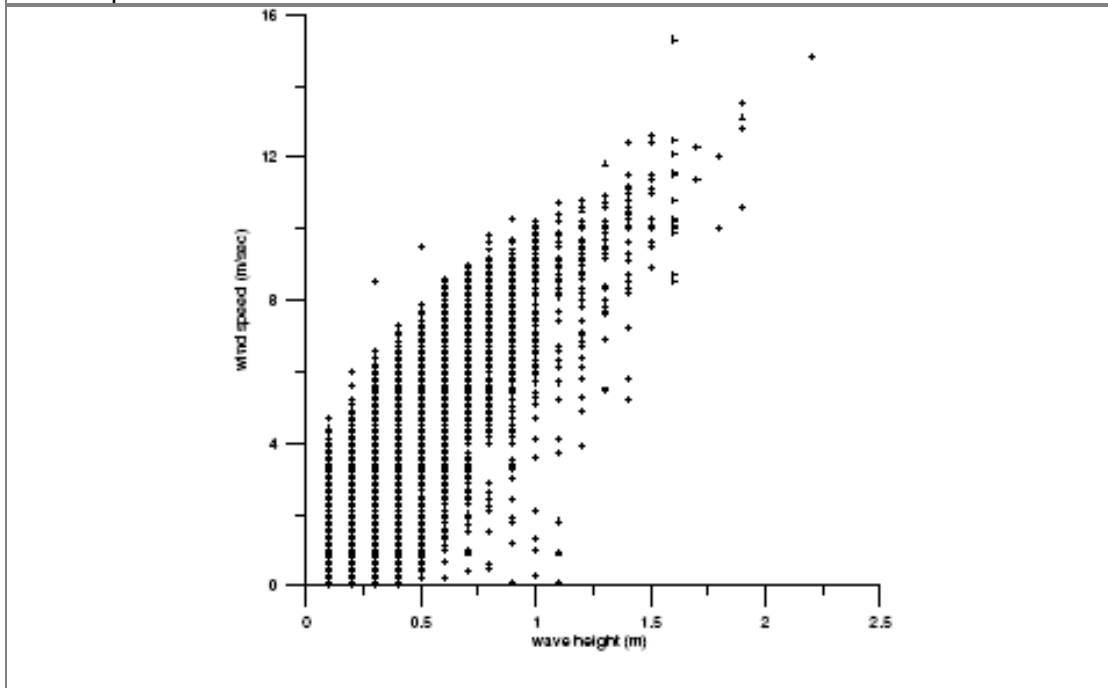
Διάγραμμα 6.26 Διάγραμμα διασποράς του σημαντικού ύψους κύματος και της ταχύτητας του ανέμου.
