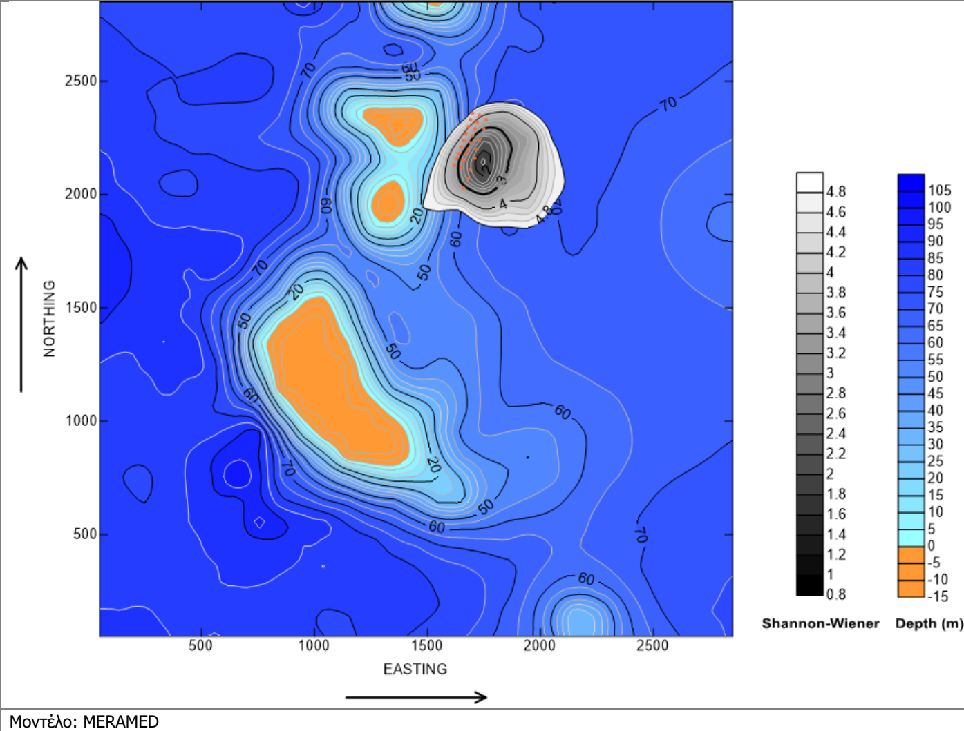
Διάγραμμα 7.104 Μεταβολή ποικιλότητας βενθικής κοινότητας (Π8 – Σενάριο 4).
