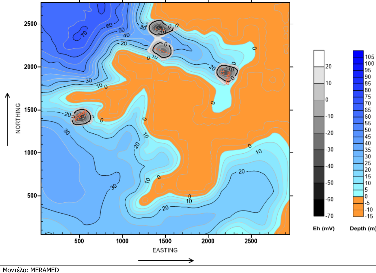
Διάγραμμα 7.45 Μεταβολή δυναμικού οξειδοαναγωγής του ιζήματος (Π5 – Σενάριο 2).
