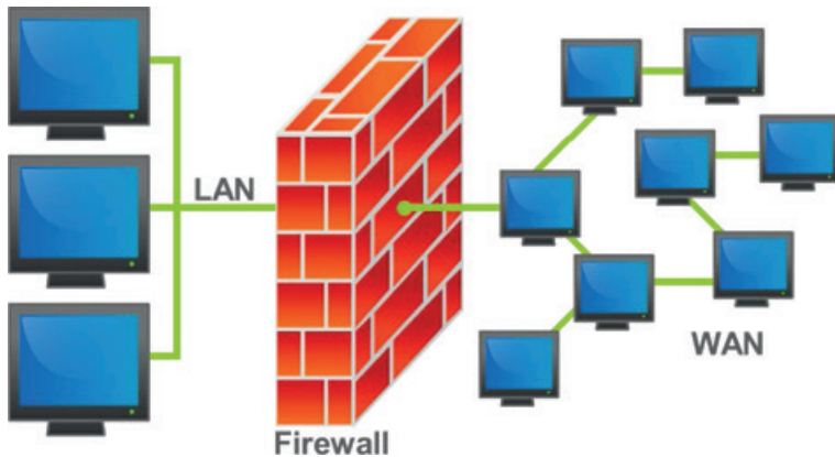
Εικόνα 8.13: Τείχος Προστασίας.
