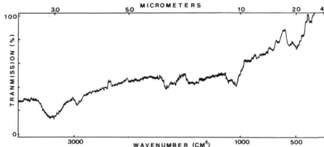
Σχήμα 1. Φάσμα απορρόφησης της υπέρυθρης ακτινοβολίας του συνδετικού υλικού της προετοιμασίας. Οι περιοχές υψηλής απορρόφησης αντιστοιχούν στις χαρακτηριστικές απορροφήσεις των πεπτιδικών δεσμών ζωικής κόλλας \nu(\text{C-N}) : 1450\text{ cm}^{-1} , \delta(\text{N-H}) : 1540\text{-}1550\text{ cm}^{-1} , \nu(\text{C=O}) : 1640\text{ cm}^{-1} , \nu(\text{N-H}) : 2940\text{ cm}^{-1} , 3400\text{ cm}^{-1} . Perkin Elmer Spectrophotometer 283.
