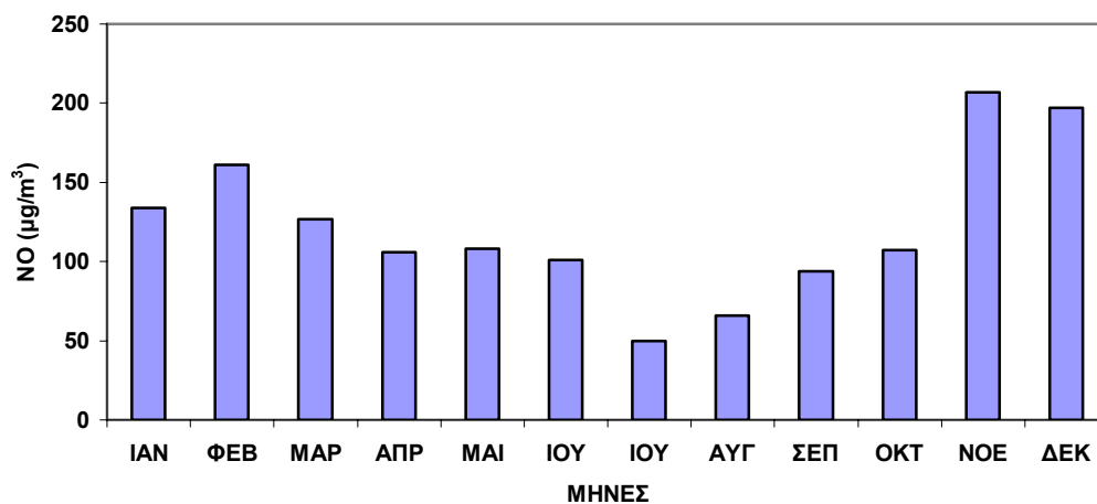
Σχήμα 2.11. Μέσες μηνιαίες τιμές NO 2 στο σταθμό Πατησίων για το έτος 2006.
