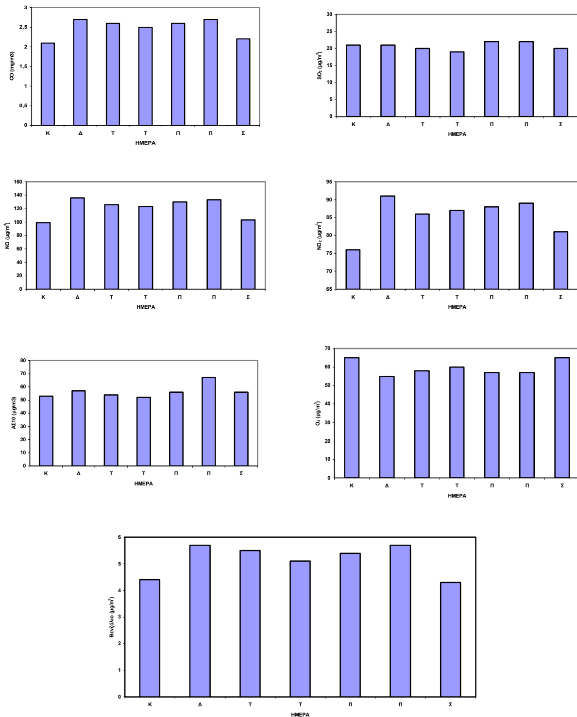
Σχήμα 2.15 Ημερήσια μεταβολή συγκεντρώσεων CO , SO 2 , NO και NO 2 στο σταθμό Πατησίων, AΣ 10 στο σταθμό Αριστοτέλους, O 3 στο σταθμό Λυκόβρυση και βενζόλιο στο σταθμό Πατησίων για το έτος 2006.
