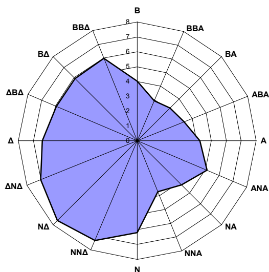
Σχήμα 3.8 Μέσες τιμές AΣ 10 (σε µg/m 3 ) για το έτος 2006 στο σταθμό Αριστοτέλους για κάθε διεύθυνση του ανέμου.
