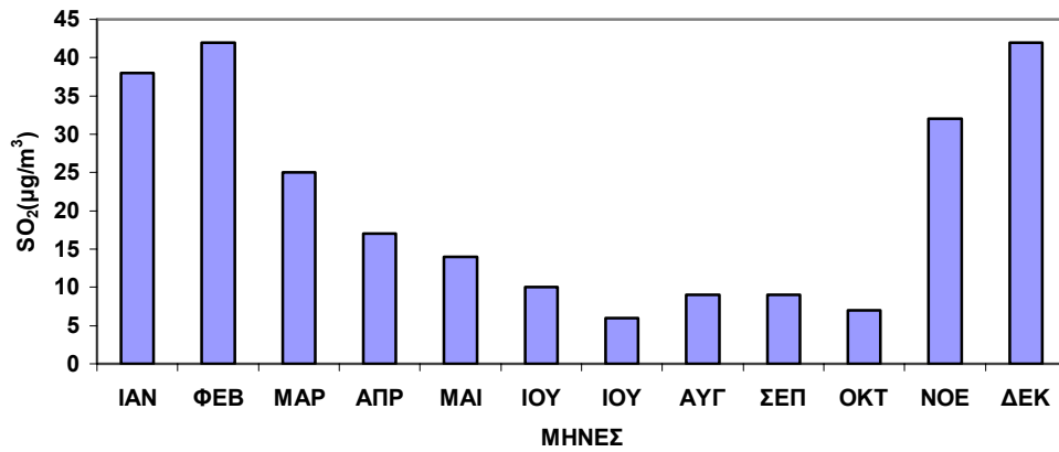
Σχήμα 2.9. Μέσες μηνιαίες τιμές SO 2 στο σταθμό Πατησίων για το έτος 2006.
