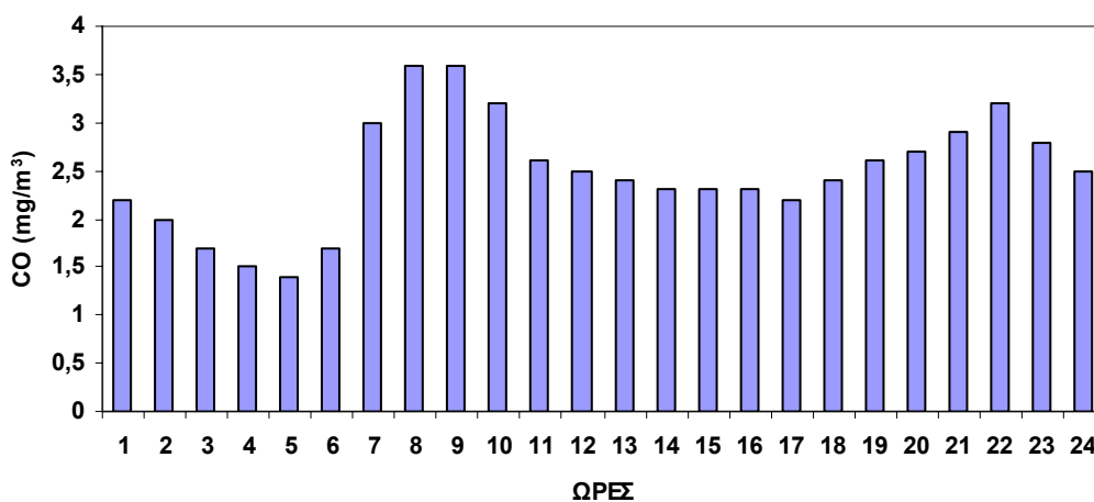
Σχήμα 2.16 Ωριαία μεταβολή CO στο σταθμό Πατησίων για το έτος 2006.
