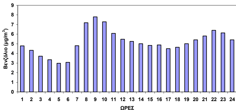
Σχήμα 2.19 Ωριαία μεταβολή βενζολίου στο σταθμό Πατησίων για το έτος 2006.
