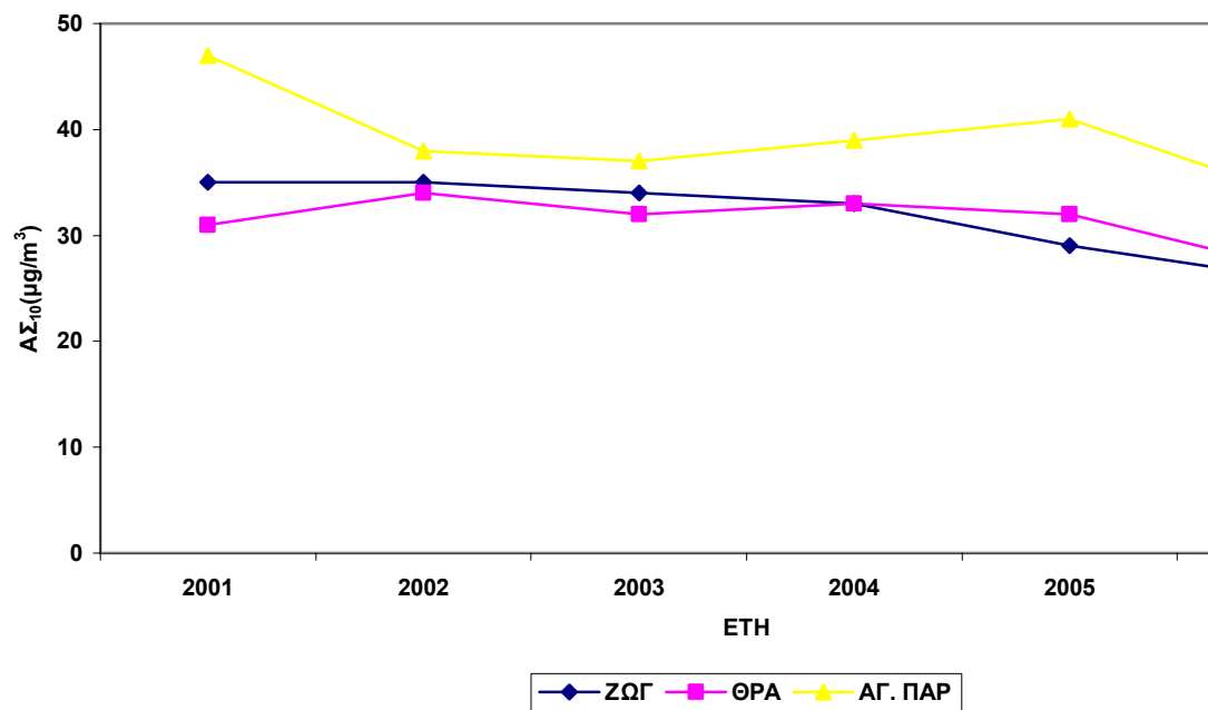
Σχήμα 2.7.β Διαχρονική μεταβολή μέσωσων ετήσιων τιμών A\Sigma_{10} , σε \mu\text{g}/\text{m}^3 .
