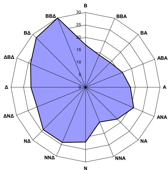
Σχήμα 3.7 Μέσες τιμές SO 2 (σε µg/m 3 ) για το έτος 2006 στο σταθμό Πατησίων για κάθε διεύθυνση του ανέμου.
