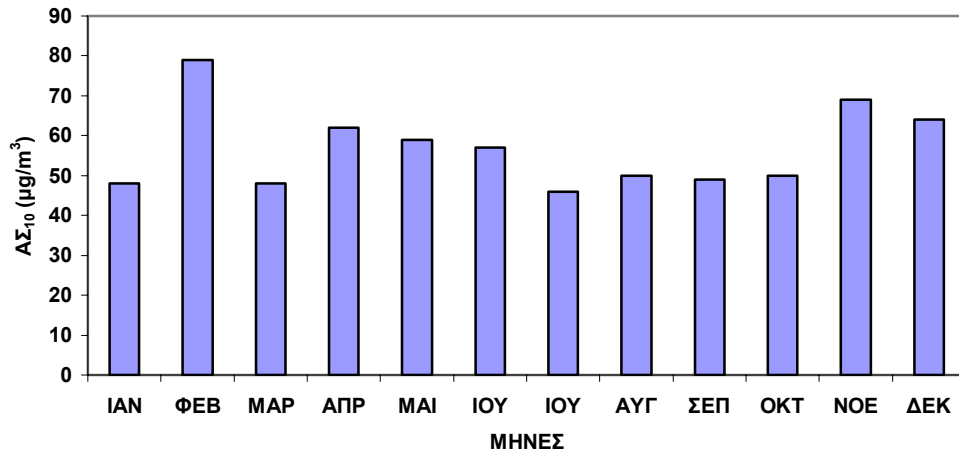
Σχήμα 2.13. Μέσες μηνιαίες τιμές ΑΣ 10 στο σταθμό Αριστοτέλους για το έτος 2006.
