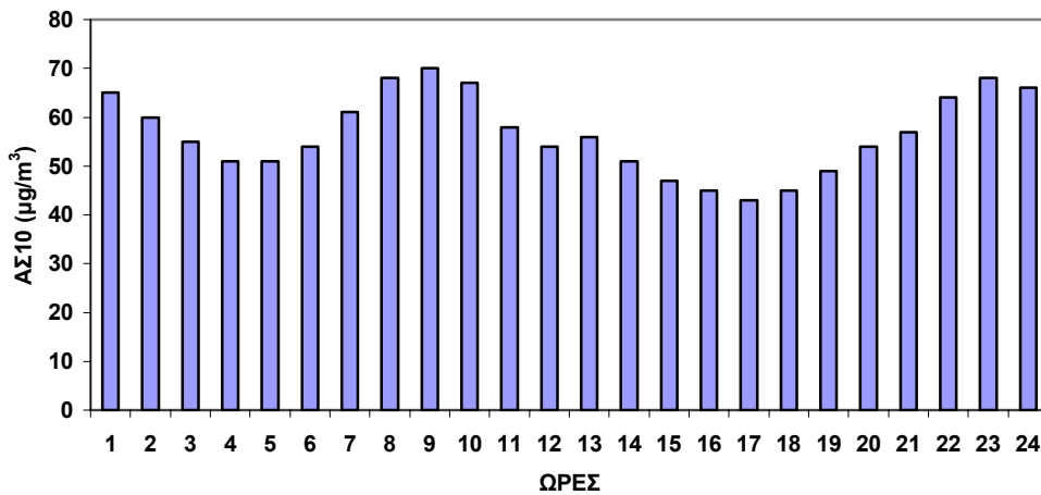
Σχήμα 2.22 Ωριαία μεταβολή ΑΣ 10 στο σταθμό Αριστοτέλους για το έτος 2006.
