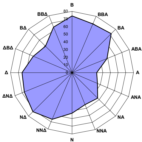
Σχήμα 3.3 Μέσες τιμές NO_2 (σε \mu g/m^3 ) για το έτος 2006 στο σταθμό Πατησίων για κάθε διεύθυνση του ανέμου.
