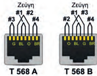
Εικόνα 2.4.1.κα: Συρμάτωση
