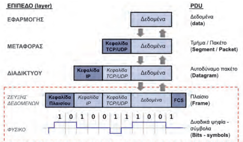
Εικόνα 1.3.α: Ενθυλάκωση
