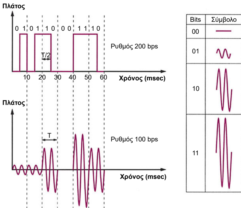
Σχήμα 2-14 Ρυθμός μετάδοσης bit διπλάσιος του ρυθμού μετάδοσης συμβόλων. Κάθε ζευγάρι bit αναπαριστάται από τις αντίστοιχες κυματομορφές του πίνακα
