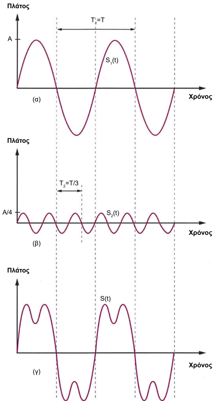
Σχήμα 2-5 Αναπαράσταση σήματος στο πεδίο του χρόνου (α) s_1(t)=\sin(2\pi ft) : ημιτονικό σήμα συχνότητας f (β) s_2(t)=\sin(2\pi(3f)t) : ημιτονικό σήμα συχνότητας 3f (γ) s(t)=\sin(2\pi ft)+\sin(2\pi(3f)t) Το σήμα s(t) είναι η σύνθεση των σημάτων s_1(t) και s_2(t)
