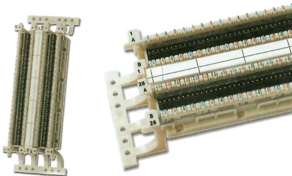
Εικόνα 5-9 Οριολωρίδα
