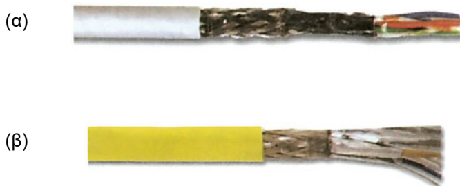
Εικόνα 4-4 (α) Καλώδιο S/FTP (β) Καλώδιο S/STP
