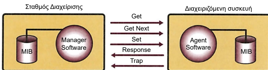
Σχήμα 8-7 Εντολές που ανταλλάσσονται στο πρότυπο διαχείρισης SNMP
