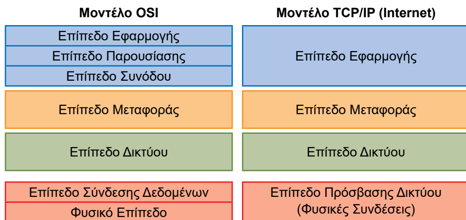
Σχήμα 7-4 Μοντέλα OSI και TCP/IP
