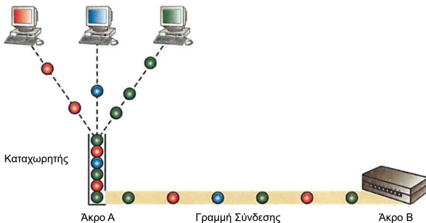
Σχήμα 1-17 Στατιστική πολυπλεξία
