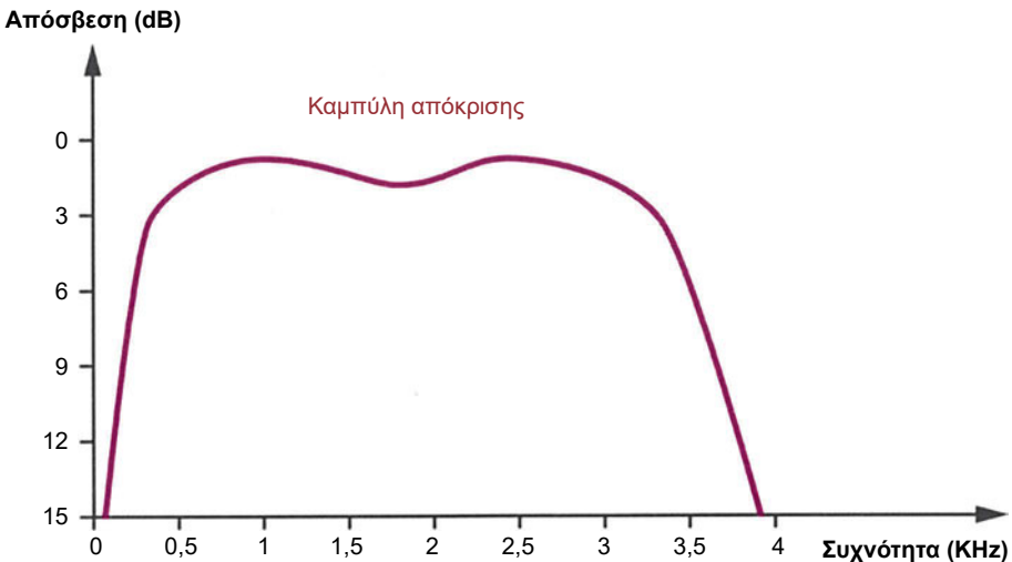
Σχήμα 3-9 Εξασθένιση σε σχέση με τη συχνότητα
