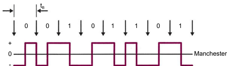
Σχήμα 4-16 Κωδικοποίηση Manchester
