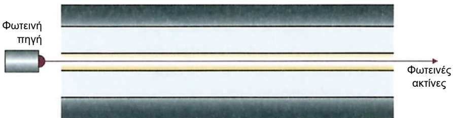
Σχήμα 4-9 Μονότροπη οπτική ίνα (single mode fiber optic)
