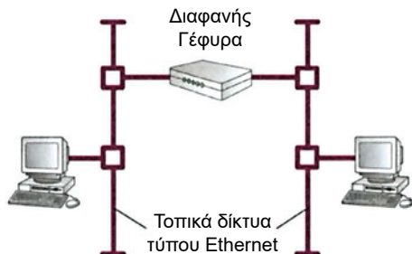
Σχήμα 5-10 Διαφανής γέφυρα
