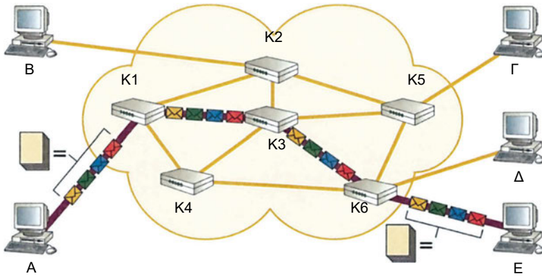
Σχήμα 1-15 Δίκτυο μεταγωγής πακέτων. Πρώθηση πακέτων με τη μέθοδο νοητού κυκλώματος
