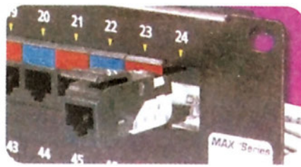
Εικόνα 5-7 Λεπτομέρεια κατανεμητή όπου φαίνεται ο IDC υποδοχέας
