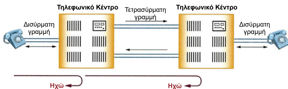
Σχήμα 3-15 Δημιουργία ηχούς
