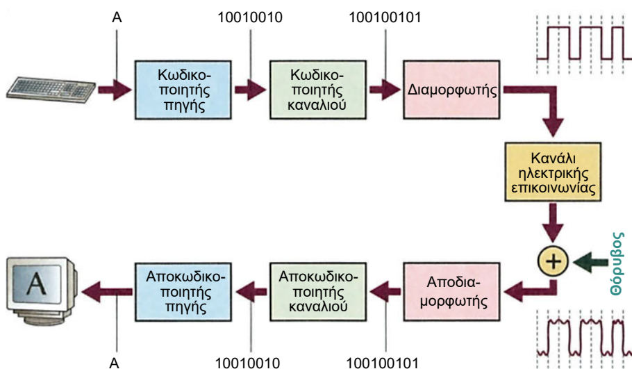
Σχήμα 2-13 Μετάδοση της εξόδου του πληκτρολογίου ενός υπολογιστή
