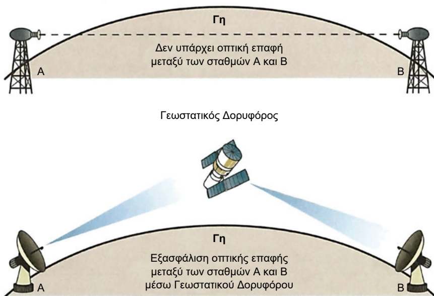
Σχήμα 3-6 Καμπυλότητα γης
