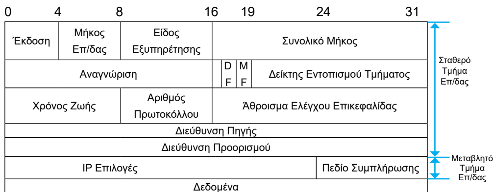
Σχήμα 7-14 IP αυτοδύναμο πακέτο
