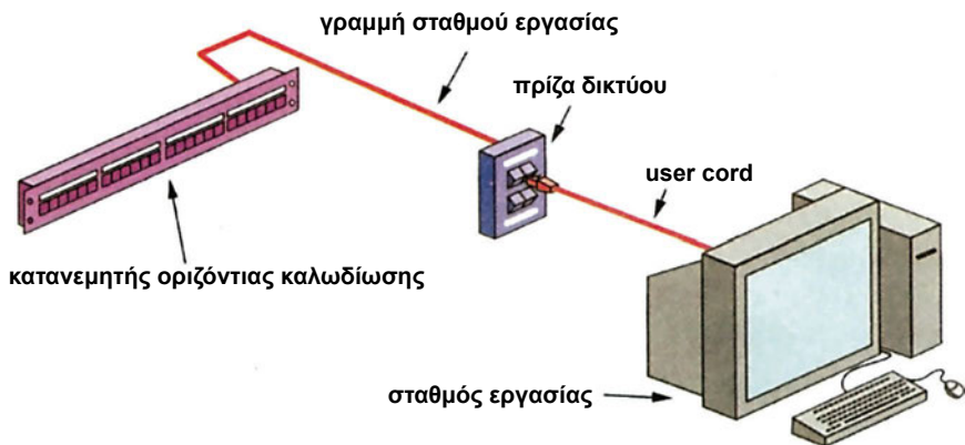
Σχήμα 5-21 Η σύνδεση σταθμών εργασίας με τον κατανεμητή οριζόντιας καλωδίωσης
