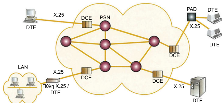
Σχήμα 6-2 Δίκτυο X.25
