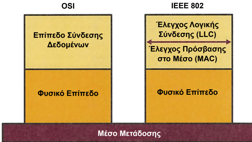
Σχήμα 4-14 Σχέση μοντέλων αναφοράς OSI και IEEE 8
